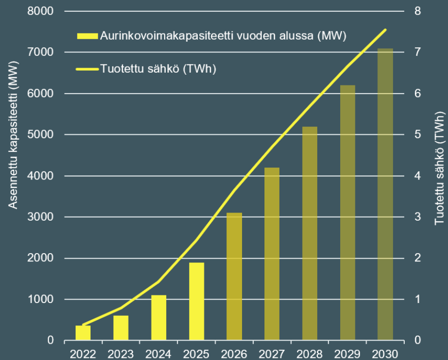
Aurinkovoimakapasiteetin kasvuennuste
